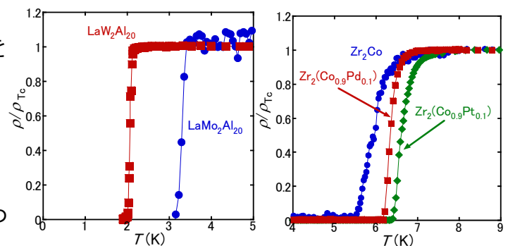
各種超伝導体の超伝導転移
